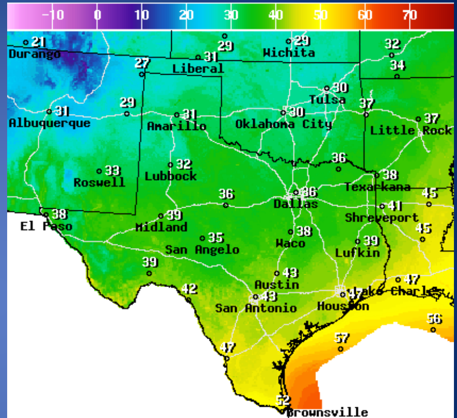
Temperature(F) For Sun Jan 28 2024 4AM EST (Sun Jan 28 2024 09Z)
