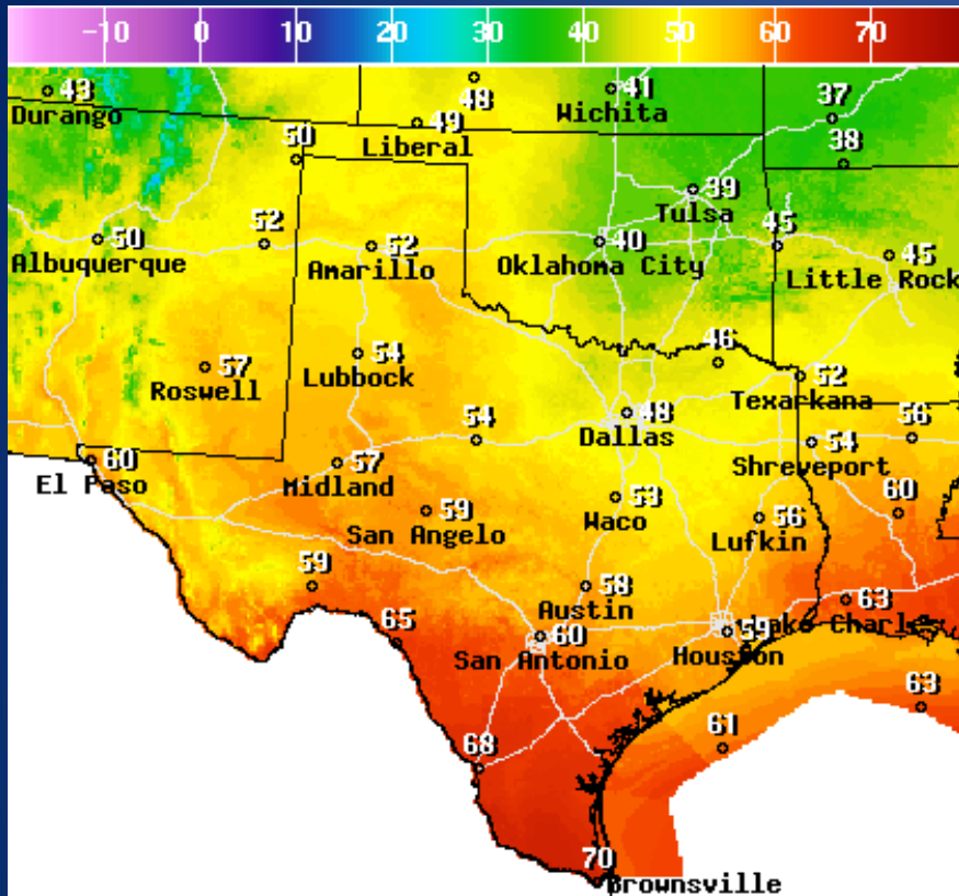
Temperature(F) For Sat Jan 27 2024 4PM EST (Sat Jan 27 2024 21Z)
