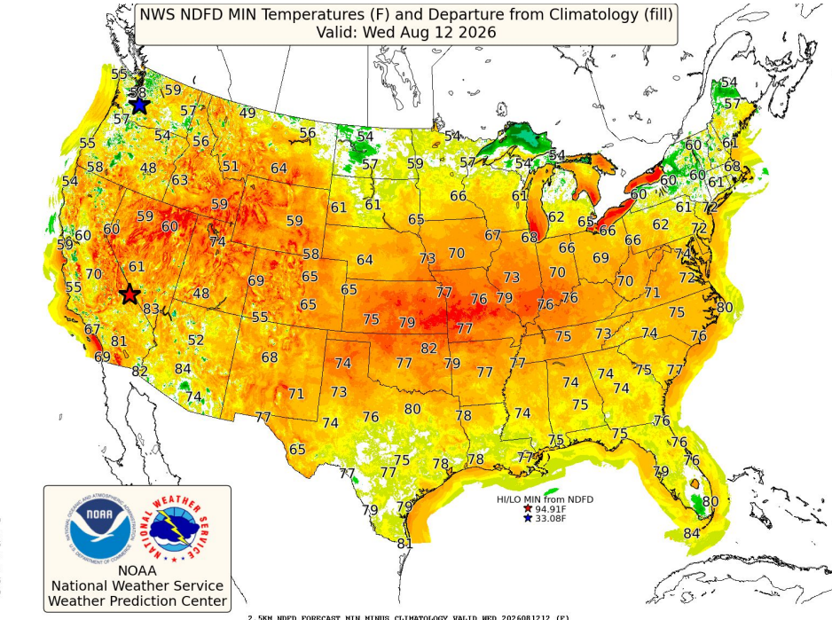
Day 3 Night
